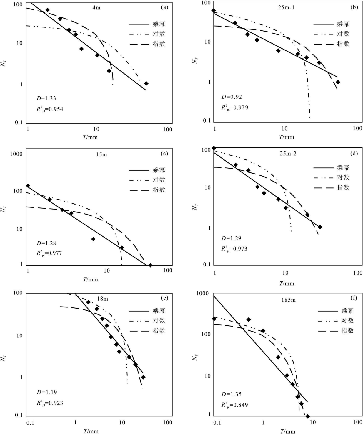
图 7 脉体宽度( T )与聚集频度数( N_T )对数图
