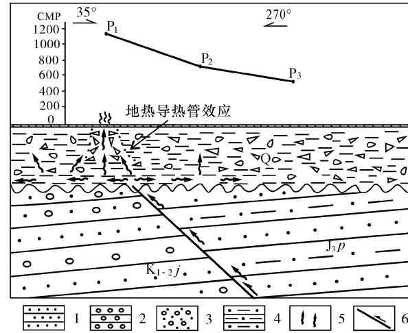
图 4 地热流近地表传导示意图
