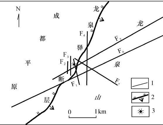
图 2 同安镇地区遥感地质解译图 Fig.2 Geological remote sensing image of the Tongan town 1. 遥感解译的断层; 2. 逆断层; 3. 地热异常位置
