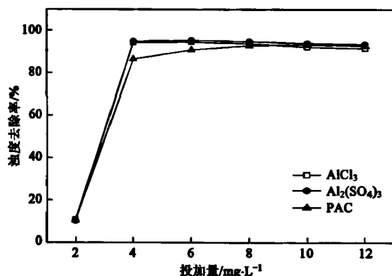
图 2 3 种混凝剂的除浊效果
