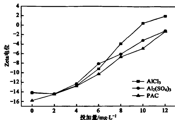
图 4 3 种混凝剂形成絮体的 Zeta 电位
