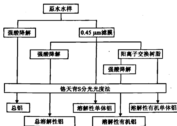
图 1 不同组分残留铝的分离流程
