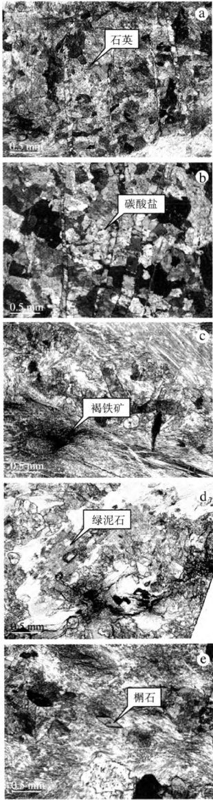
图 3 样品中的次要矿物 Fig. 3 Auxiliary minerals in sample a. 石英 +; b. 碳酸盐 +; c. 褐铁矿 +; d. 绿泥石 -; e. 榍石 +
